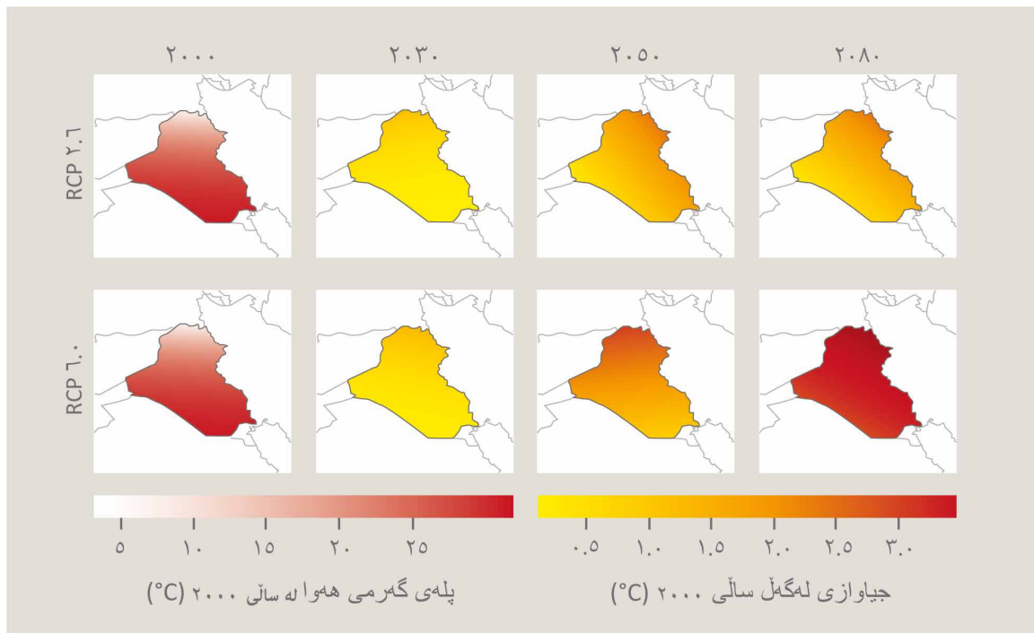
وهسفرکردنی نهخشه یه دووهم: دوو پیشبینی پلهی گهرمی ههوا له عێراق بۆ سیناریۆ جیاوازهکانی دهردانی گازی گهرمخانهیی (گۆرانکاری ناوچهیی) ۱۹ .
