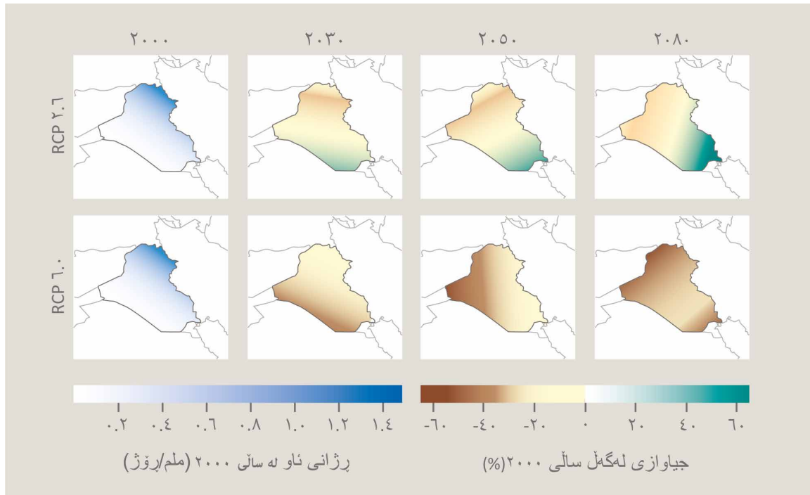
وهسفرکردنی نهخشه یه کهم: تیکرای پیشبینی بارانبارینی سالانه له عێراق بۆ سیناریۆ جیاوازهکانی دهردانی گازی گهرمخانهیی، به بهراورد به سالی ۲۰۰۰ (گۆرانکاریه ناوچهییهکان) ۱۸ .
